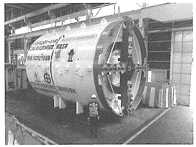
シールドマシンは、貯留管を築造する際に地下を掘り進める機械で、全重量は約220t、ジャンボジェット機本体（約160t）の1.4倍となります。
