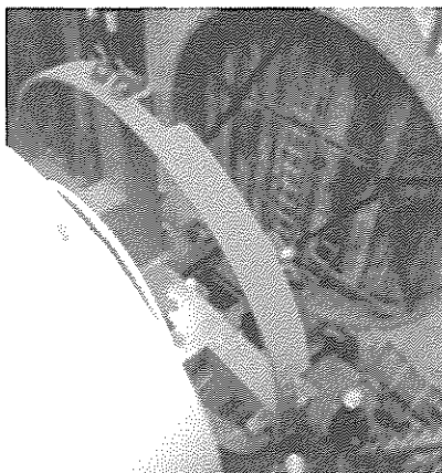
立坑内でのシールドマシン組み立て状況（R 2.11） 立坑は、地下約 17 m 掘り下げています
