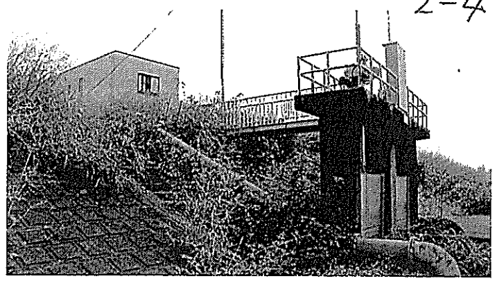
●里ポンプ場(小風)から新芝川への排水管と水門
