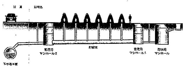
マンホールトイレ概要図
