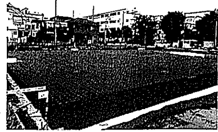
建設中のプラスチック製雨水貯留施設 (柳崎公園)
